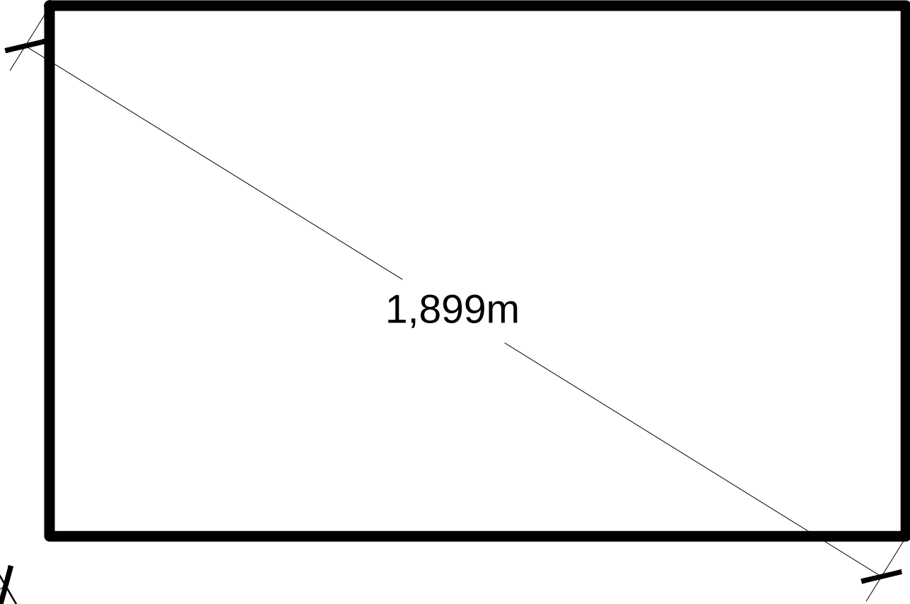
Retângulo de Ouro
