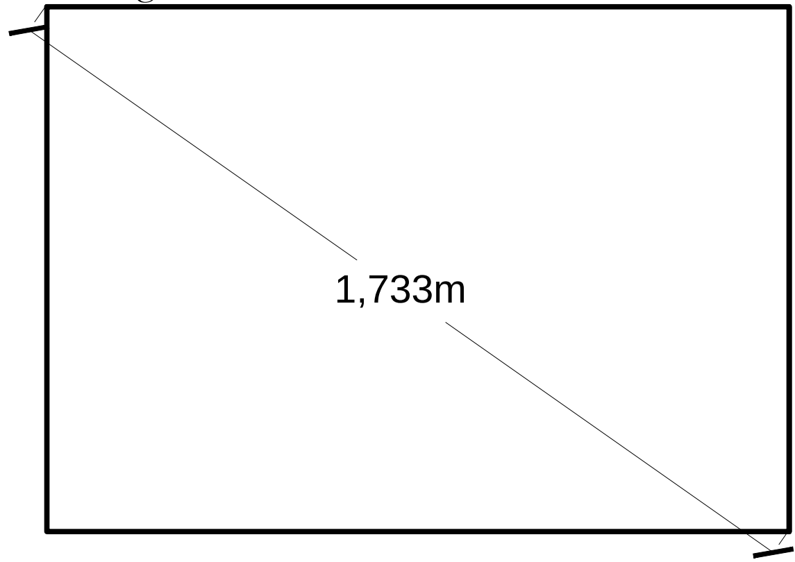
Retângulo raiz de 2
